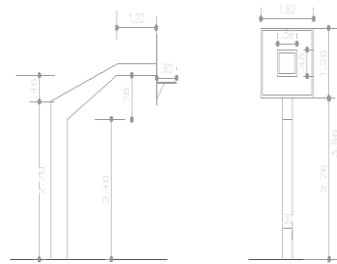
SOPORTE DE TABLERO
