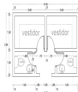
PLANTA VESTIDORES Y BAÑOS 1:75
